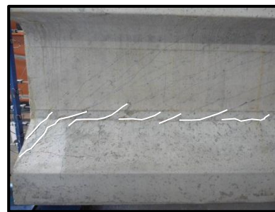
(D) Horizontal shear in Tx46
