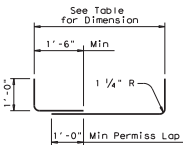
BARS D1-5 (#4)
