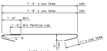
BARS Y (#4)
