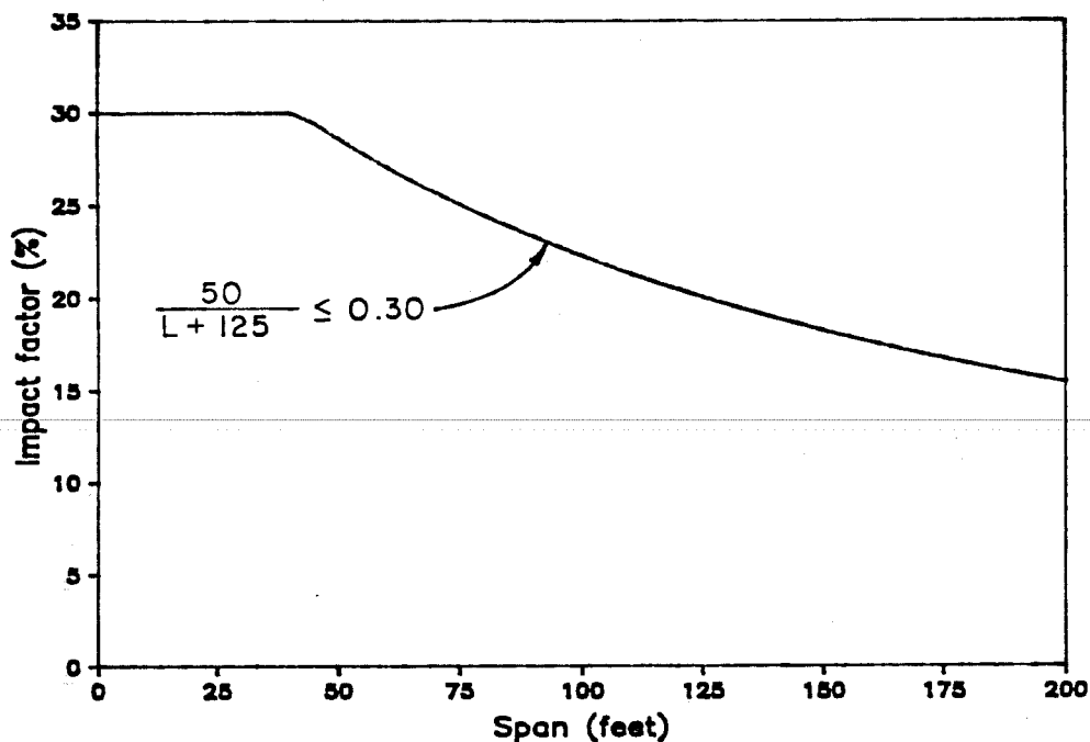
Fig. 4.28 AASHTO live load impact factor
