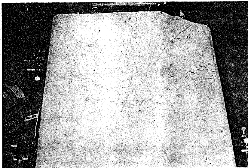
(d) Cracking at failure
