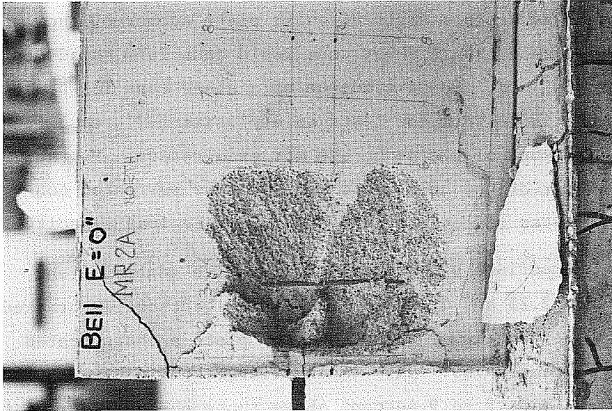
(d) Explosive failure of north side
