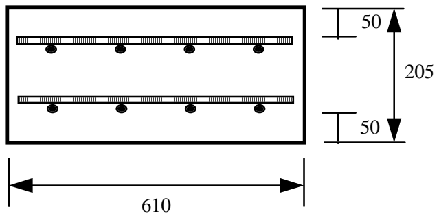
b) Side Elevation
