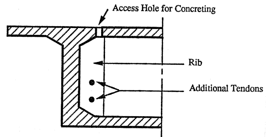
b) Rib Deviator
